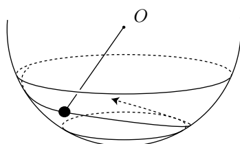
FIGURE 6. Pendule sphérique
