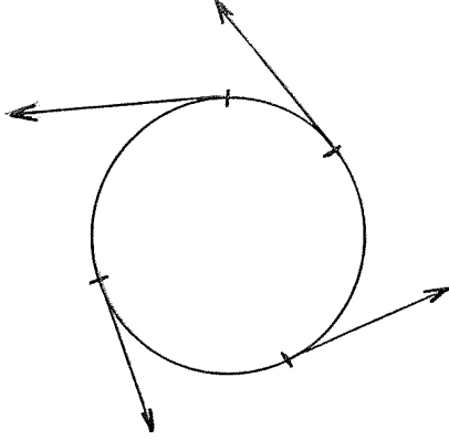
Le cercle : on peut trouver un champ de vecteurs tangents non nuls.
