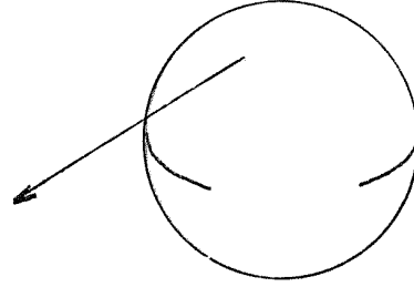
La sphère : on ne peut PAS trouver un champ de vecteurs tangents non nuls (théorème de la sphère chevelue).
