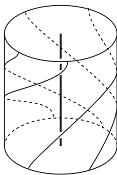
FIGURE 1. Un fibré de Seifert
