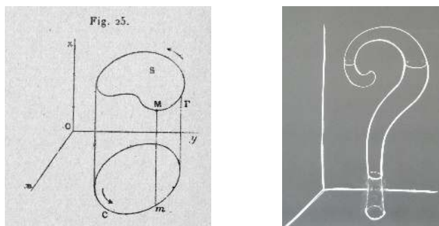
FIGURE 17. Interrogation sur la validité de la formule de Stokes
