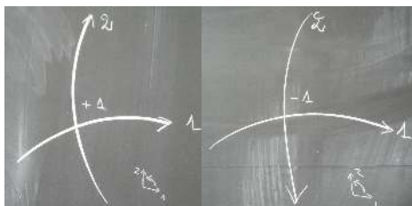
FIGURE 15. Nombre d'intersection local, au tableau
