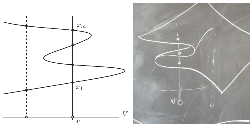
FIGURE 10. L'image inverse d'un point général
