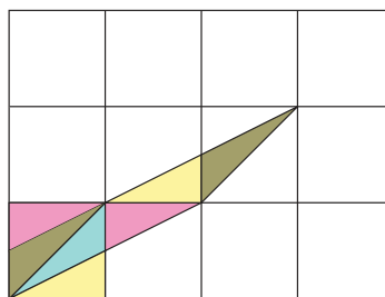
FIGURE 12. Une application de degré 1
